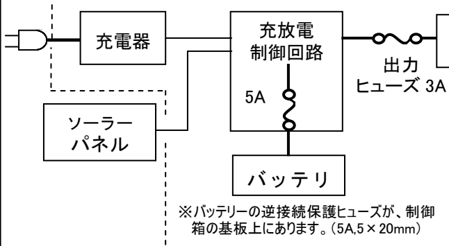
バッテリーボックス内部図
