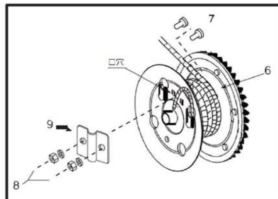
図3:ケーブル設置
